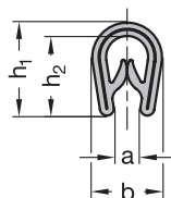
Profilquerschnitt bei
